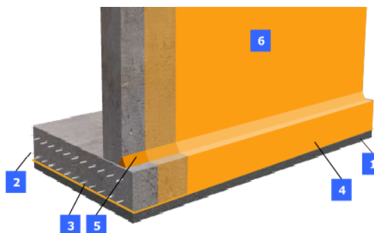
Rys 1. Klin przyścienny z zewnątrz wraz z innymi elementami uszczelnienia: 1-chudy beton; 2-zbrojenie; 3-płyta fundamentowa; 3-warstwa Hydrostopu-Mieszanki równomiernie rozsypana; 4-bok płyty uszczelniony Hydrostopem-Mieszanką Profesjonalną ; 5-klin z Hydrostopu-Zaprawy Wodoszczelnej ; 6-bok ściany uszczelniony Hydrostopem-Mieszanką Profesjonalną .
